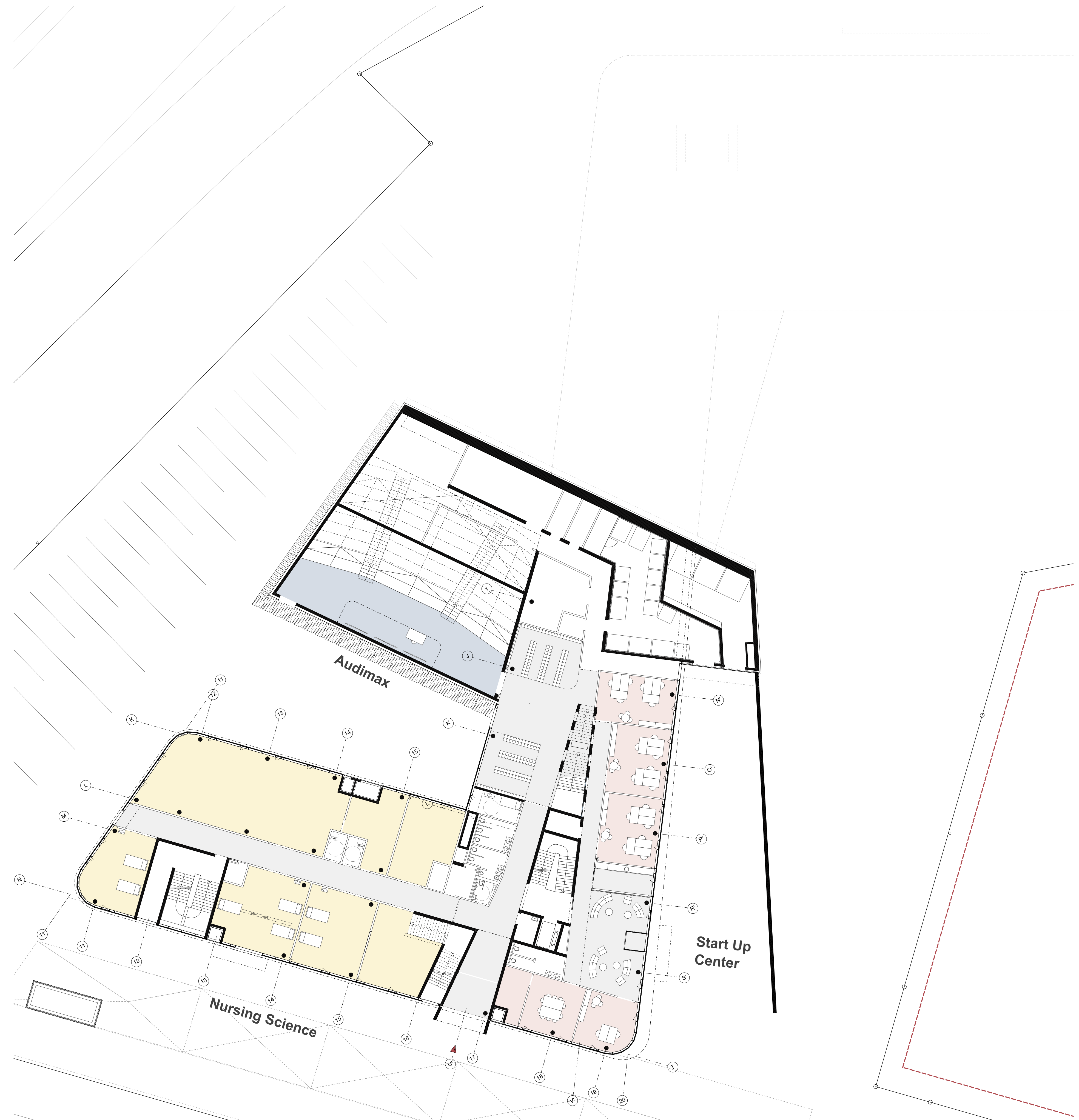
Grundriss -1 Sockel M1:200
