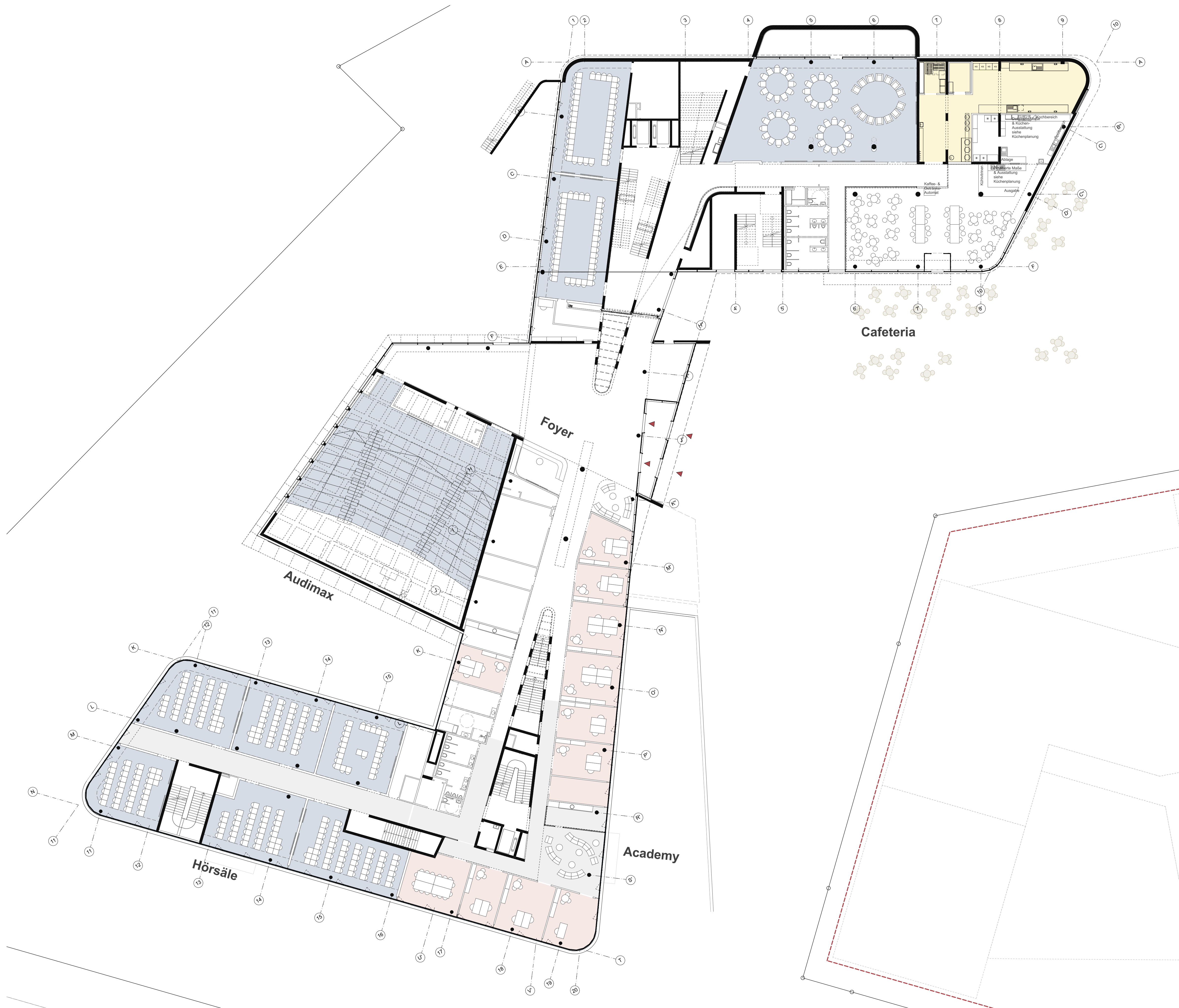
Grundriss EG M1:200
